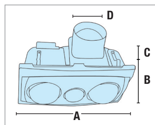
▶ Dimensions - Classic Heat 'n Vent
